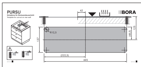
Obr. 10.22 Šablona pro výřez zadní stěny
