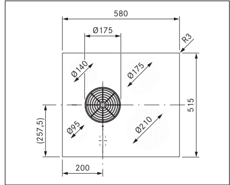
Obr. 3.4 Rozměry spotřebiče PURSU – pohled shora
