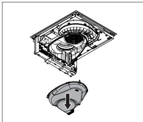
Obr. 10.37 Demontáž spodní části sací komory
