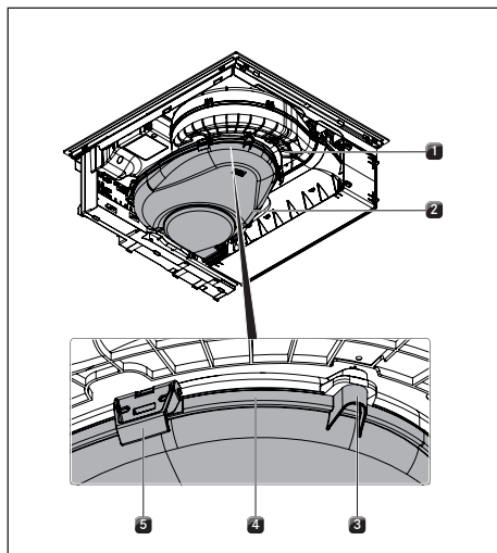
Obr. 8.3 Skříň ventilace
