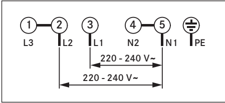
Obr. 10.39 Schéma připojení u dvoufázové přípojky
