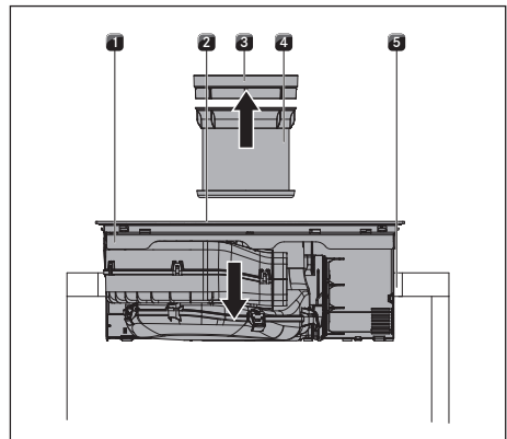
Obr. 10.12 Nasazení varné desky
