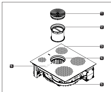
Obr. 5.1 Varná deska
