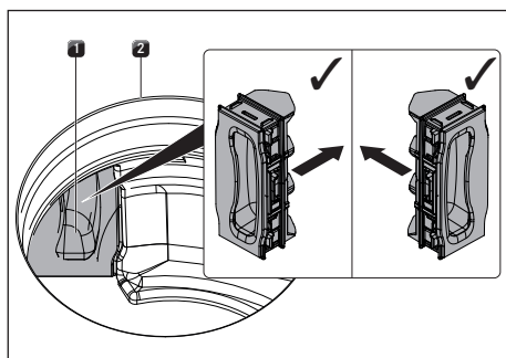
Obr. 8.10 Nasazení výměnné klapky filtru
