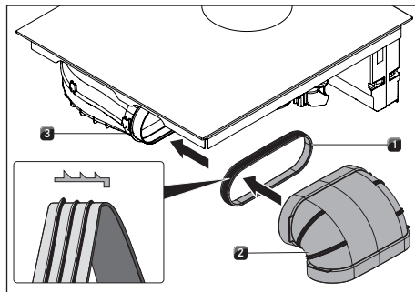
Obr. 10.16 Připojení systému odťahových potrubí
