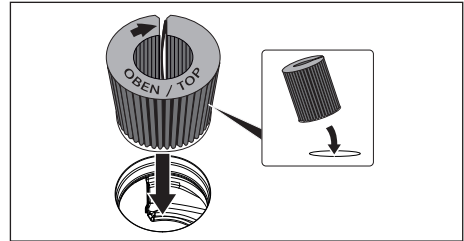
Obr. 10.33 Nasazení filtru s aktivním uhlím do otvoru odsavače
