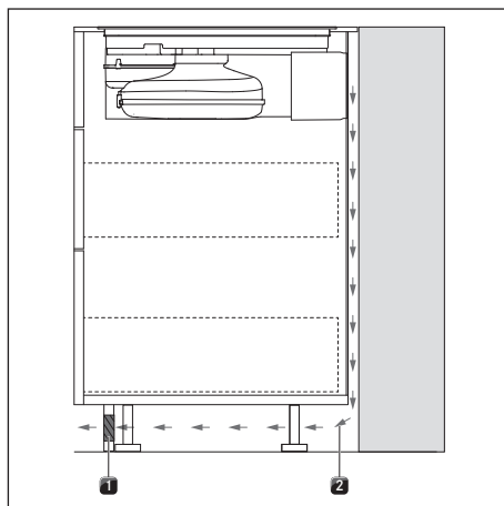
Obr. 10.17 Otvor na zpětné proudění vzduchu v oblasti soklu
