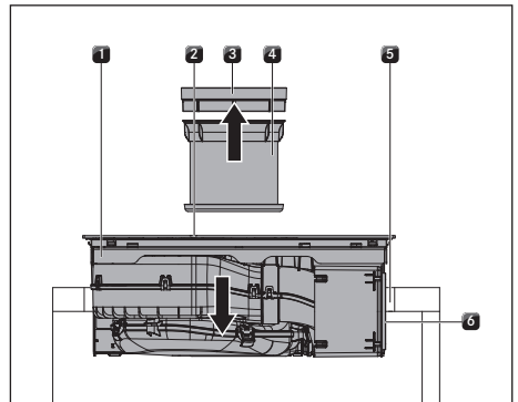
Obr. 10.26 Upevnění varné desky do středu
