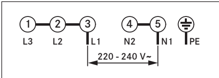
Obr. 10.40 Schéma připojení u jednofázové přípojky
