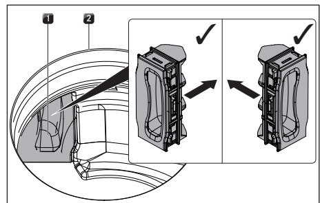
Obr. 10.35 Nasazení výměnné klapky filtru
