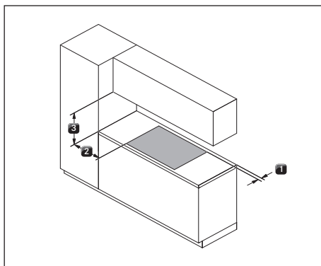
Obr. 10.3 předepsané bezpečnostní odstupy
