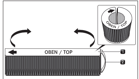
Obr. 8.7 Filtr s aktivním uhlím
