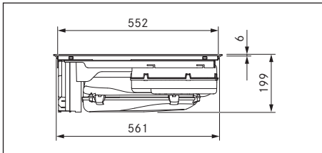
Obr. 3.2 Rozměry spotřebiče PURSA – pohled zepředu
