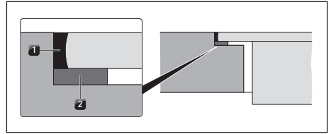
Obr. 10.25 Těsnicí páska při plošně zarovnané montáži
