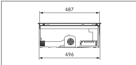
Obr. 3.3 Rozměry spotřebiče PURSA – pohled z boku
