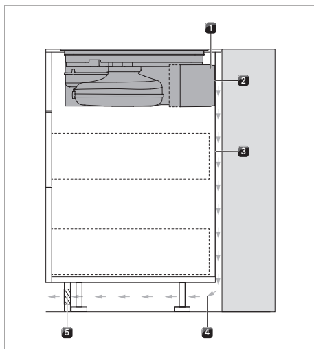
Obr. 10.18 Varianta montáže s průchozí zadní stěnou
