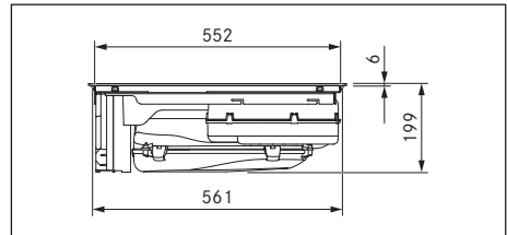
Obr. 3.5 Rozměry spotřebiče PURSU – pohled zepředu
