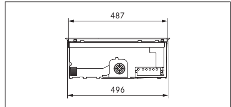
Obr. 3.6 Rozměry spotřebiče PURSU – pohled z boku
