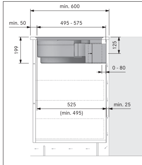
Obr. 10.20 Rozměry montáže u recirkulujícího vzduchu, varianta montáže A
