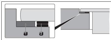
Obr. 10.15 Podložky k nastavení výšky
