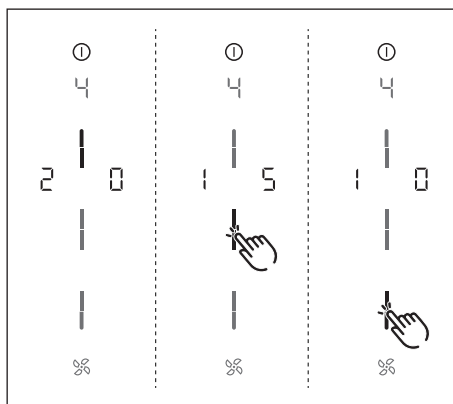
Obr. 7.4 Položka nabídky 4: Doba provozu dojezdové automatiky
