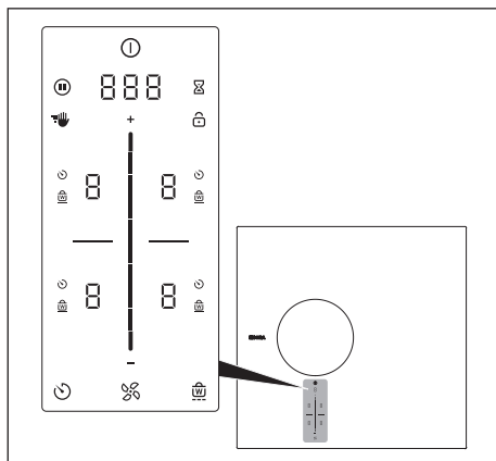
Obr. 5.4 Centrální dotykový ovládací panel s posuvníkem
