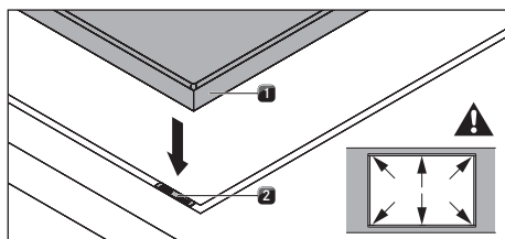
Obr. 10.14 Vložení podložky k nastavení výšky
