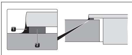
Obr. 10.10 Těsnicí páska při montáži na povrch
