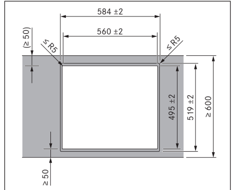
Obr. 10.5 Rozměry výřezu pro plošně zarovnanou montáž
