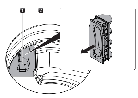
Obr. 8.4 Sejmутí výměnné klapky filtru
