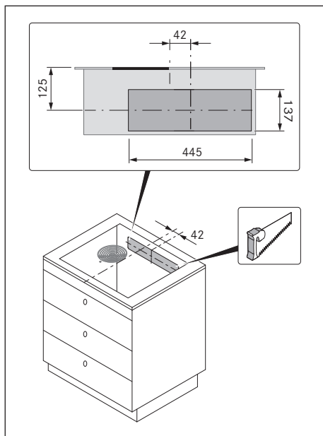
Obr. 10.21 Výřez v zadní stěně
