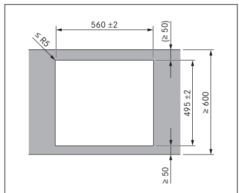
Obr. 10.7 Rozměry výřezu pro montáž na povrch
