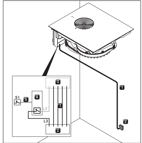
Obr. 10.42 Schéma zapojení s externím spínacím kontaktem
