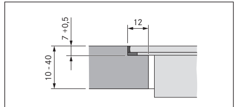
Obr. 10.6 Rozměr drážky pro plošně zarovnanou montáž
