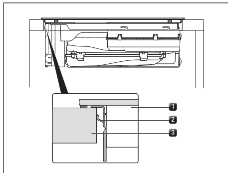
Obr. 10.27 Upevnění varné desky
