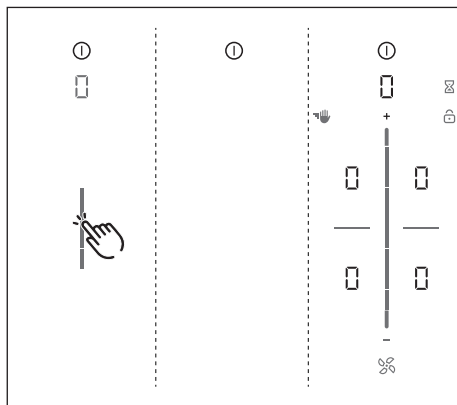
Obr. 7.11 Položka nabídky 0: Tovární nastavení
