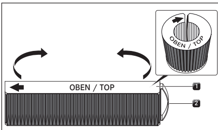
Obr. 10.32 Filtr s aktivním uhlím
