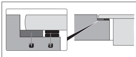
Obr. 10.29 Podložky k nastavení výšky
