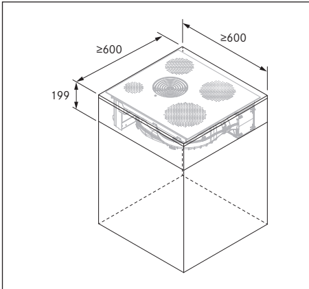
Obr. 10.4 Minimální rozměry nábytku – S Pure
