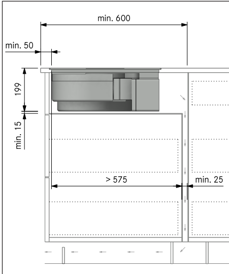
Obr. 10.23 Rozměry montáže u varianty montáže B, hloubka pracovní desky 600 mm
