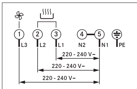
Obr. 10.38 Schéma připojení u trojfázové přípojky
