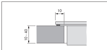
Obr. 10.8 Rozměry podkladu pro montáž na povrch
