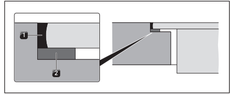
Obr. 10.11 Těsnicí páska při plošně zarovnané montáži
