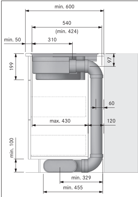
Obr. 10.9 Rozměry montáže při odtahu ven, hloubka pracovní desky 600 mm
