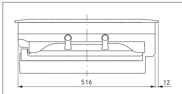
Obr. 3.7 Rozměry spotřebiče PKAS - boční pohled
