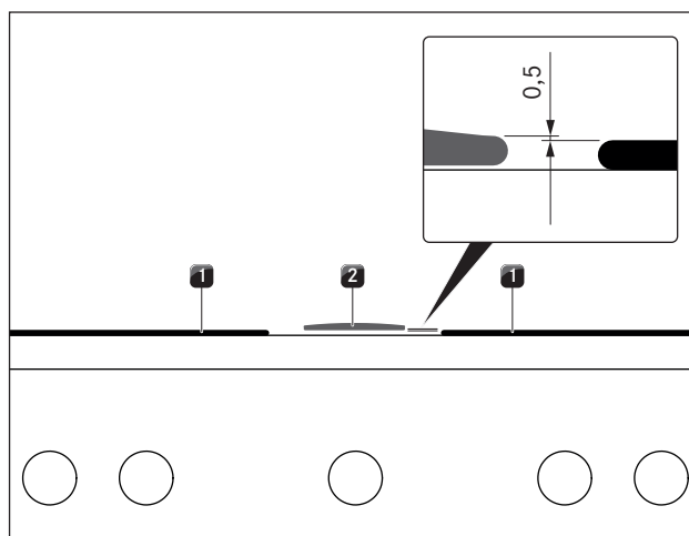
Obr. 6.11 Montáž digestoře
