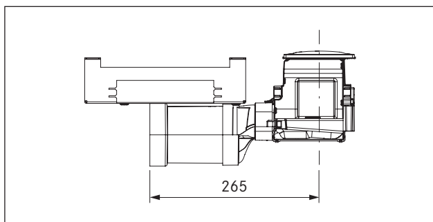
Obr. 6.18 Připojovací rozměry potrubí PKA pomocí přímého kusu
