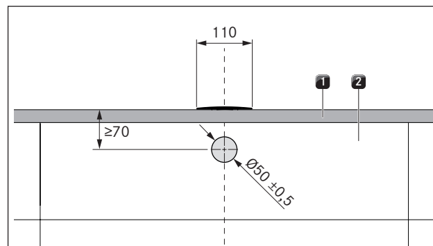
Obr. 6.20 Vrtné schéma
