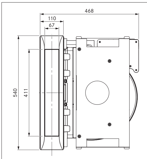
Obr. 3.5 Rozměry spotřebiče PKAS - pohled shora
