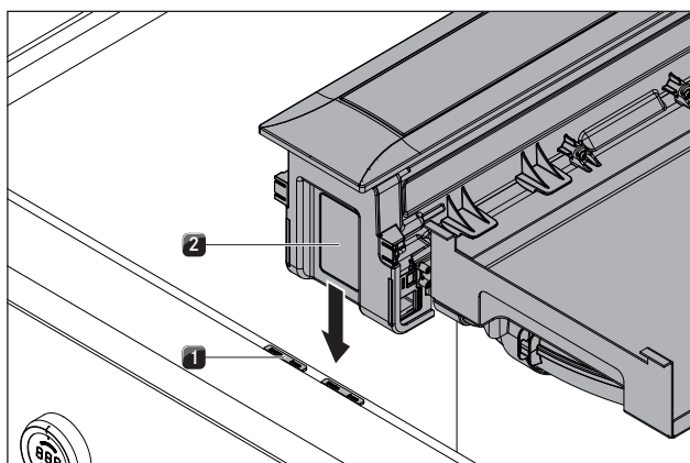
Obr. 6.10 Podložky na nastavení výšky
