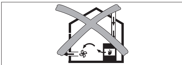
Obr. 6.36 Montáž odtahového potrubí – nepřipustné
