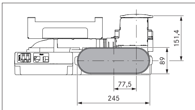
Obr. 6.19 Připojovací rozměry potrubí PKAS
