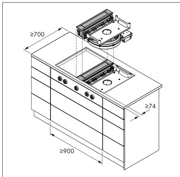
Obr. 6.8 Montážní rozměry spotřebičů PKA a PKAS
