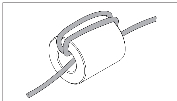
Obr. 6.40 Trojitě omotání feritového jádra připojovacím kabelem
