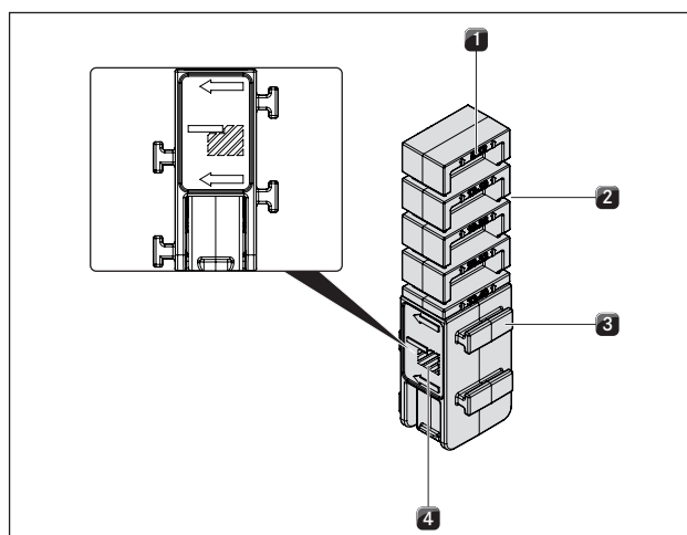
Obr. 6.12 Montážní svorka, pravá strana (plošně zarovnaná montáž)
