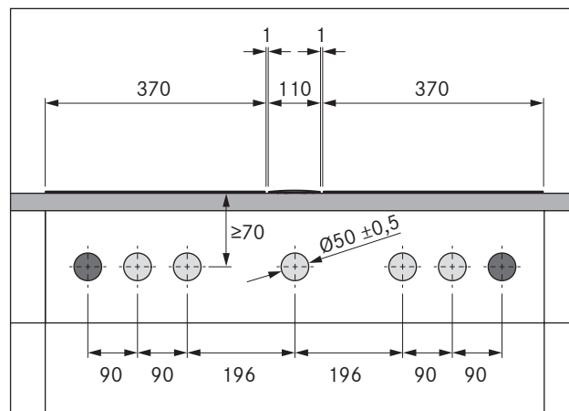
Obr. 6.21 Otvory v desce pro 2 varné desky, 2 zásuvky a 1 digestoř
