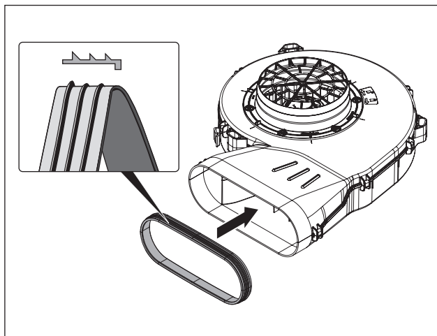
Abb. 6.21 Pozice těsnicí pásky pro montáž s přechodovým kusem (plochý kanál)
