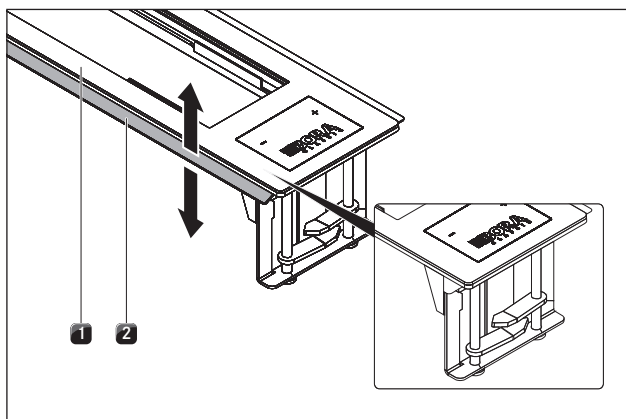
Abb. 6.13 Příprava rámu digestoře
