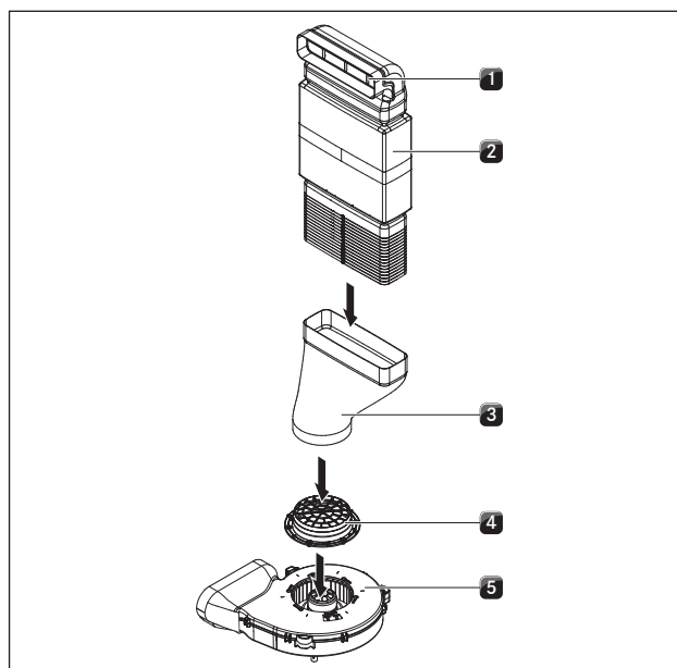
Abb. 6.18 Montáž
