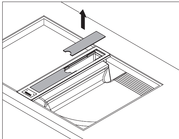
Abb. 8.1 Odstranění krytů
