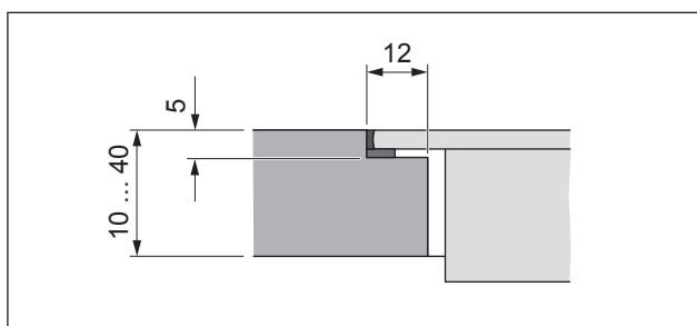
Abb. 6.3 Řez rozměr drážky
