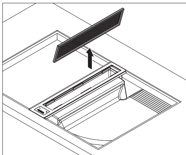
Abb. 8.2 Demontáž tukového filtru z nerezové oceli
