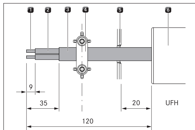
Abb. 6.31 Délky odizolace a montážní pozice připojovacího kabelu v řídicí jednotce
