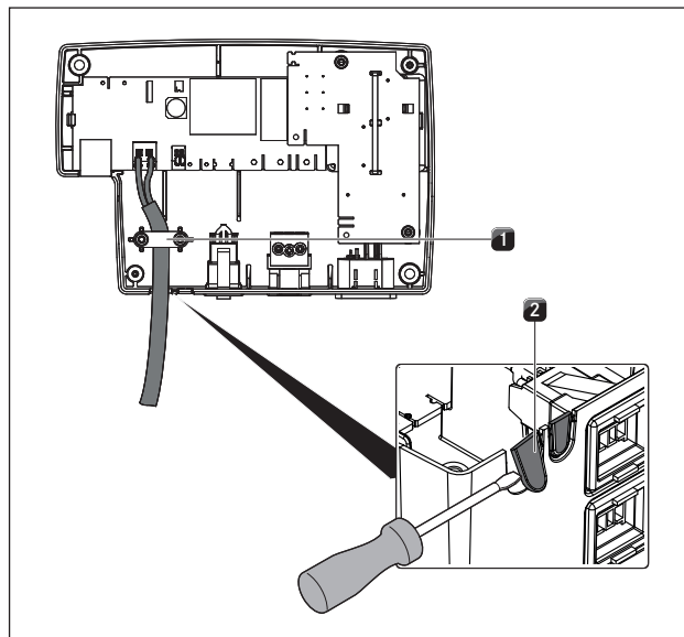
Abb. 6.33 Propojení Home-Out s odlehčením v tahu
