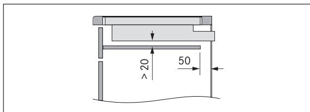
Abb. 6.8 Boční pohled na ochranu kabelu a větrání
