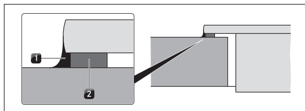
Abb. 6.7 Těsnicí páska při montáži na povrch
