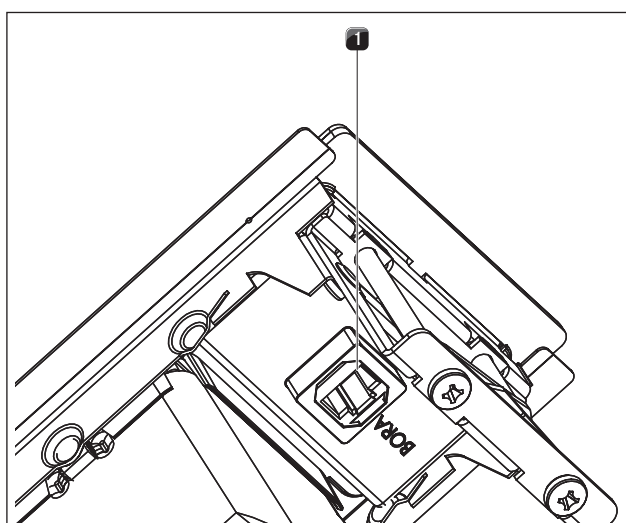
Abb. 6.27 Připojení komunikačního kabelu CAT 5
