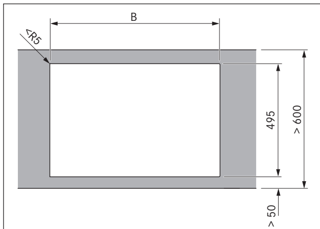
Abb. 6.4 Montáž na povrch
