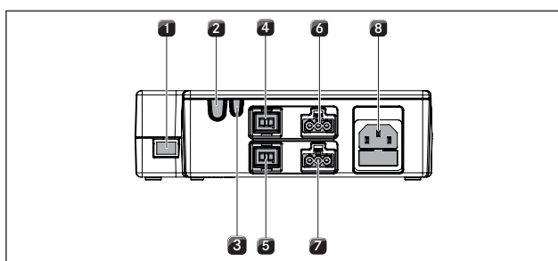
Abb. 6.26 Připojky řídicí jednotky
