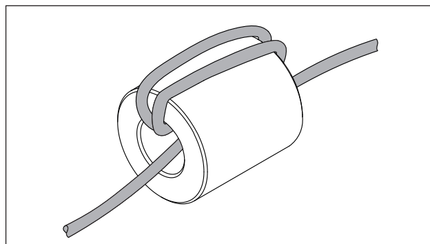
Abb. 6.30 Trojitě omotání feritové dutinky připojovacím kabelem
