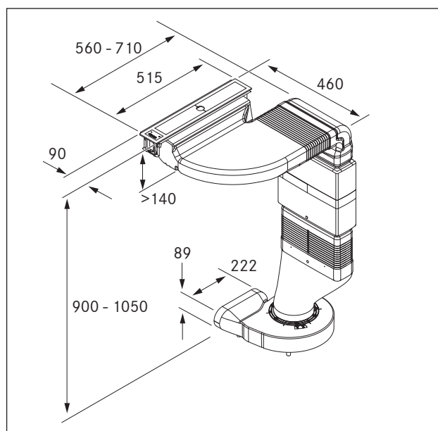
Abb. 6.9 Rozměry spotřebiče se zaobleným přechodovým kusem
