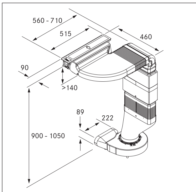
Abb. 3.1 Rozměry přístroje
