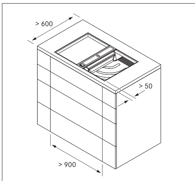
Abb. 6.12 Montážní rozměry spotřebiče
