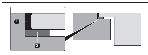
Abb. 6.6 Těsnicí páska při plošně zarovnané montáži
