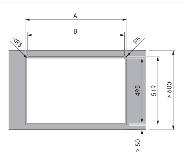
Abb. 6.2 Plošně zarovnaná montáž
