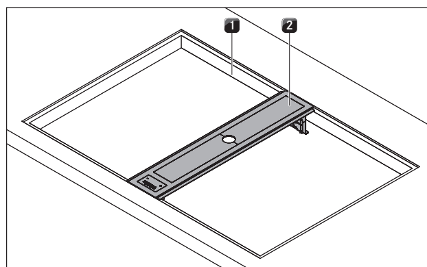
Abb. 6.14 Montáž digestoře
