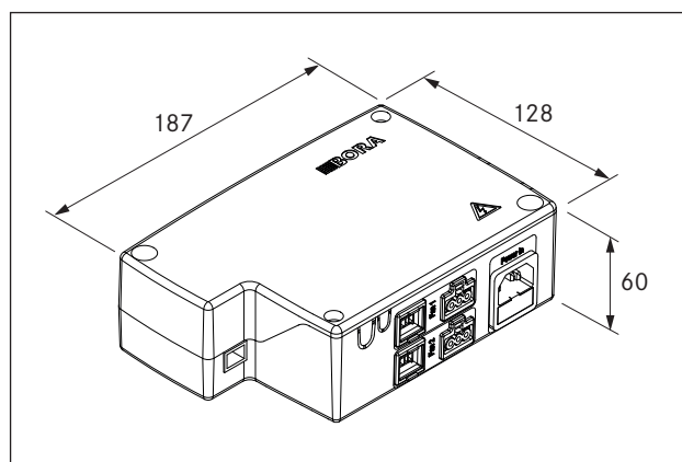
Abb. 6.11 Montážní rozměry řídicí jednotky
