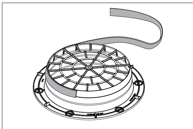
Abb. 6.20 Pozice těsnicí pásky pro montáž s trubicou kruhového průřezu
