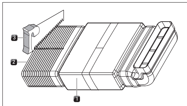
Abb. 6.17 Zkrácení modulu Silence
