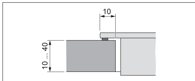
Abb. 6.5 Řez montáže na povrch
