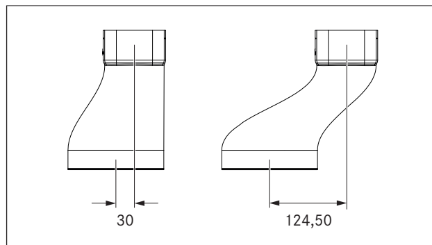
Abb. 6.10 Přesazení s přechodovými kusy
