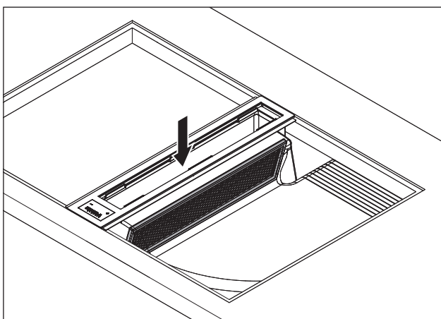
Abb. 8.3 Nasazení tukového filtru z nerezové oceli
