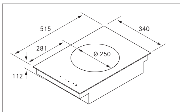
Obr. 3.1 Rozměr přístroje
