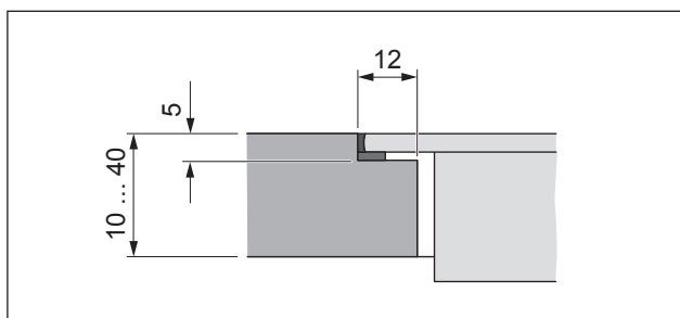
Obr. 5.3 Řez rozměr drážky
