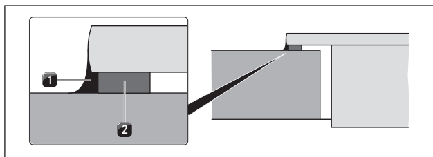
Obr. 5.7 Těsnicí páska při montáži na povrch
