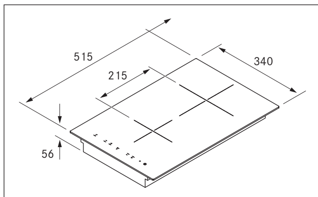
Obr. 3.1 Rozměry přístroje
