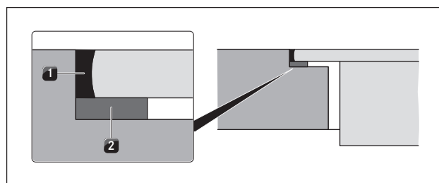
Abb. 6.7 Těsnící páska při plošně zarovnané montáži
