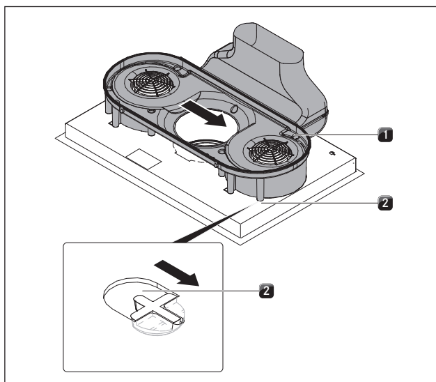
Abb. 6.32 Zacsunutí jednotky vedení vzduchu
