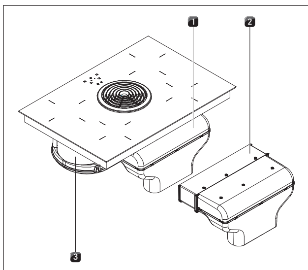
Abb. 5.3 Digestoř s odvodem vzduchu (BHA)
