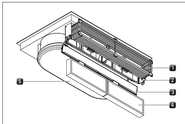
Abb. 5.2 Digestoř s recirkulací (BHU)
